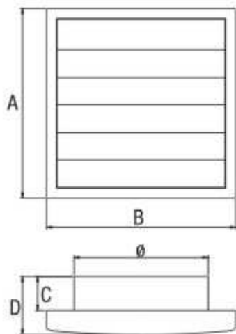
Typ Spádová mriežka B-15
