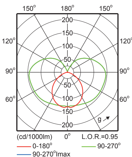
TCH128 1xTL5-21W HF
