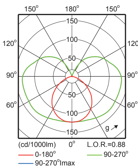
TCH128 1xTL5-14W HF
